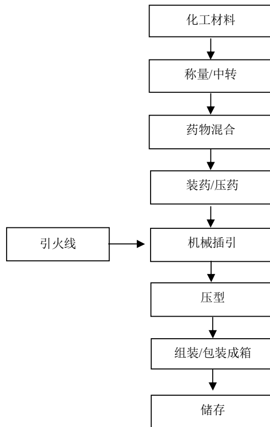
图 2-3：旋转类（彩菊）生产工艺流程图
