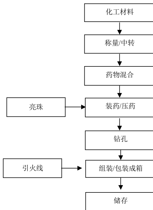
图 2-4：旋转类（大地花开）生产工艺流程图
