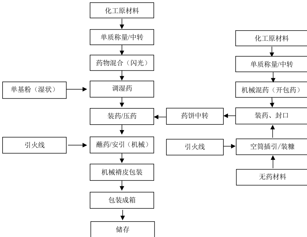
图 2-2：喷花类（闪光炮）生产工艺流程图
