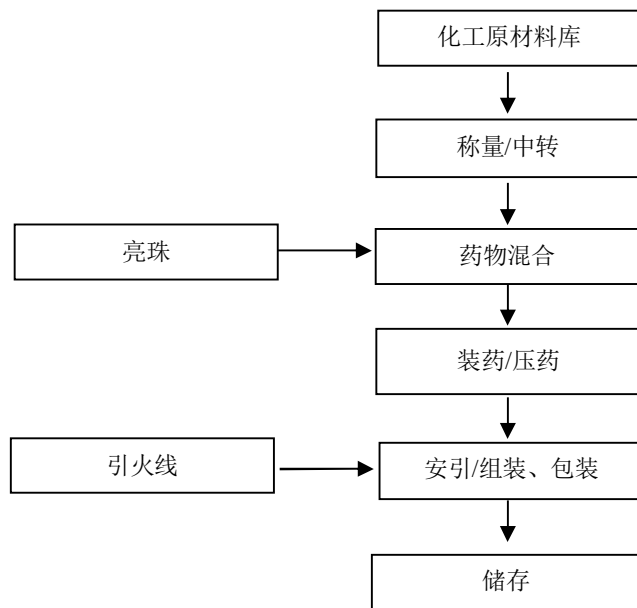
图 2-1：喷花类（花筒）产品生产工艺流程图
