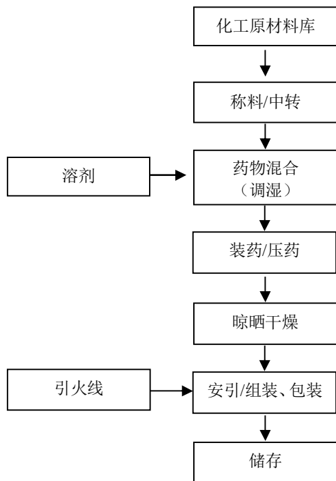
图 2-6: 玩具类（玩具造型）生产工艺流程图
