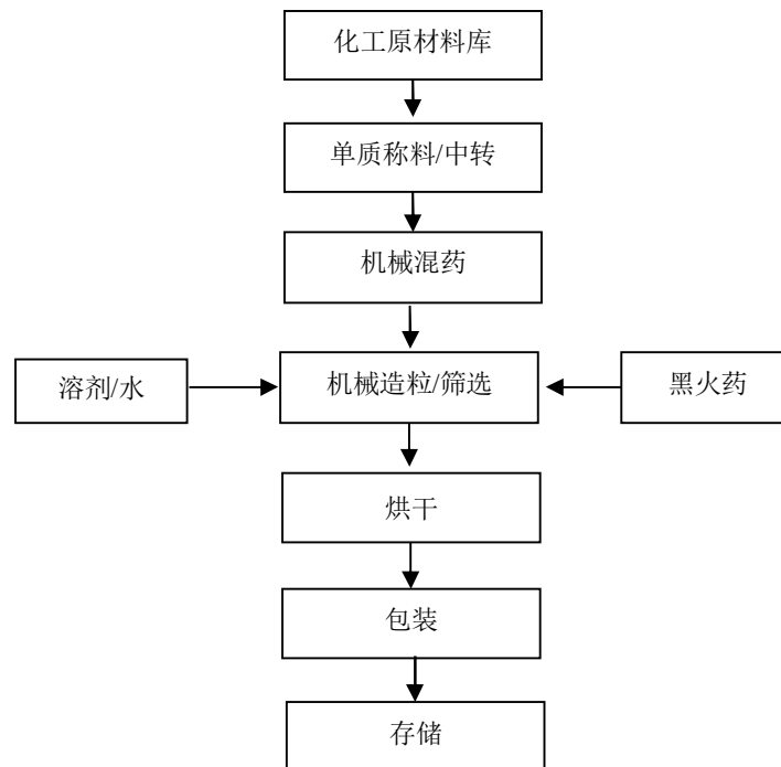
图 2-9: 亮珠生产工艺流程图
