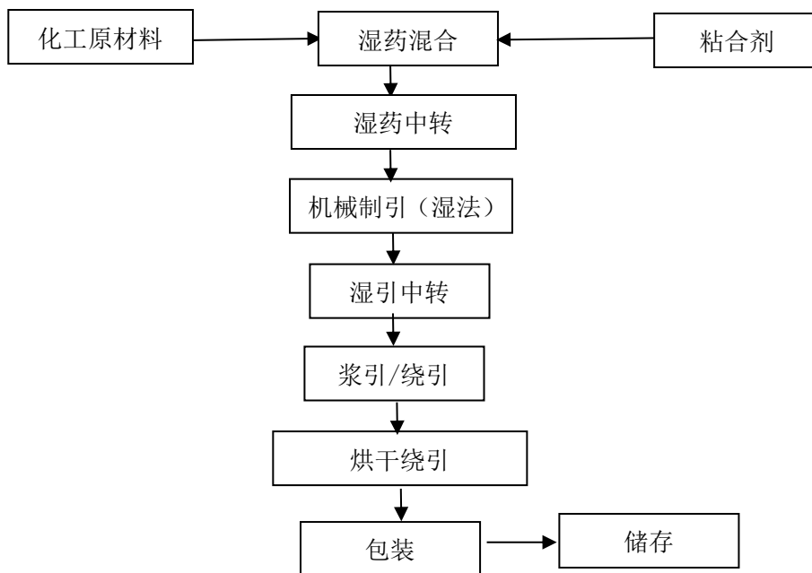
图 2-4-2 皮纸引生产工艺流程图
