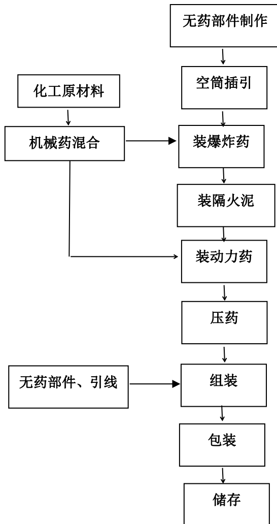
图 2-4-1 升空类（双响炮）生产流程图
