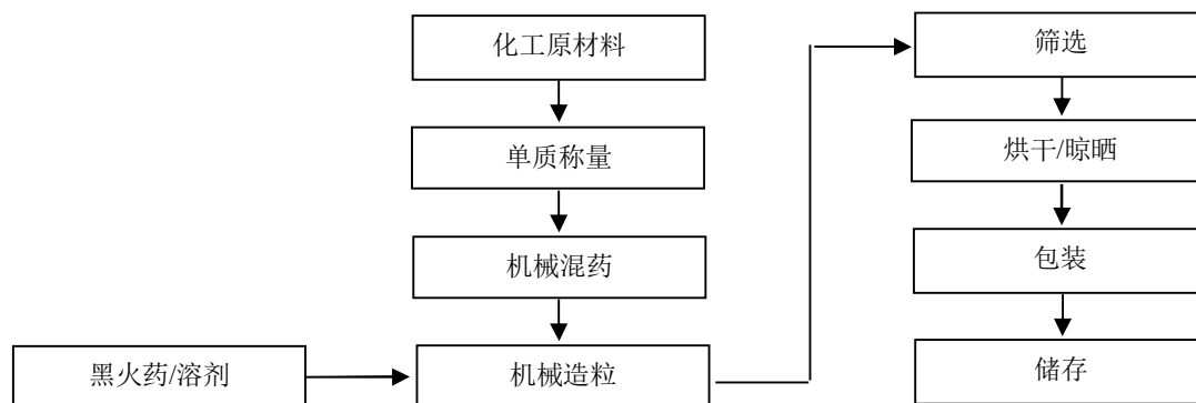
图 2-6：亮珠生产工艺流程图
