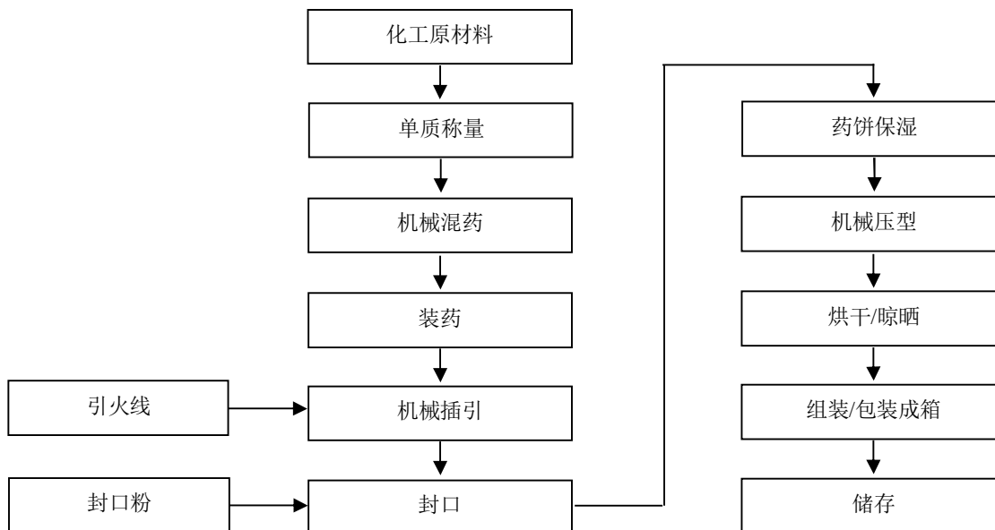
图 2-4：旋转类（彩菊）生产工艺流程图
