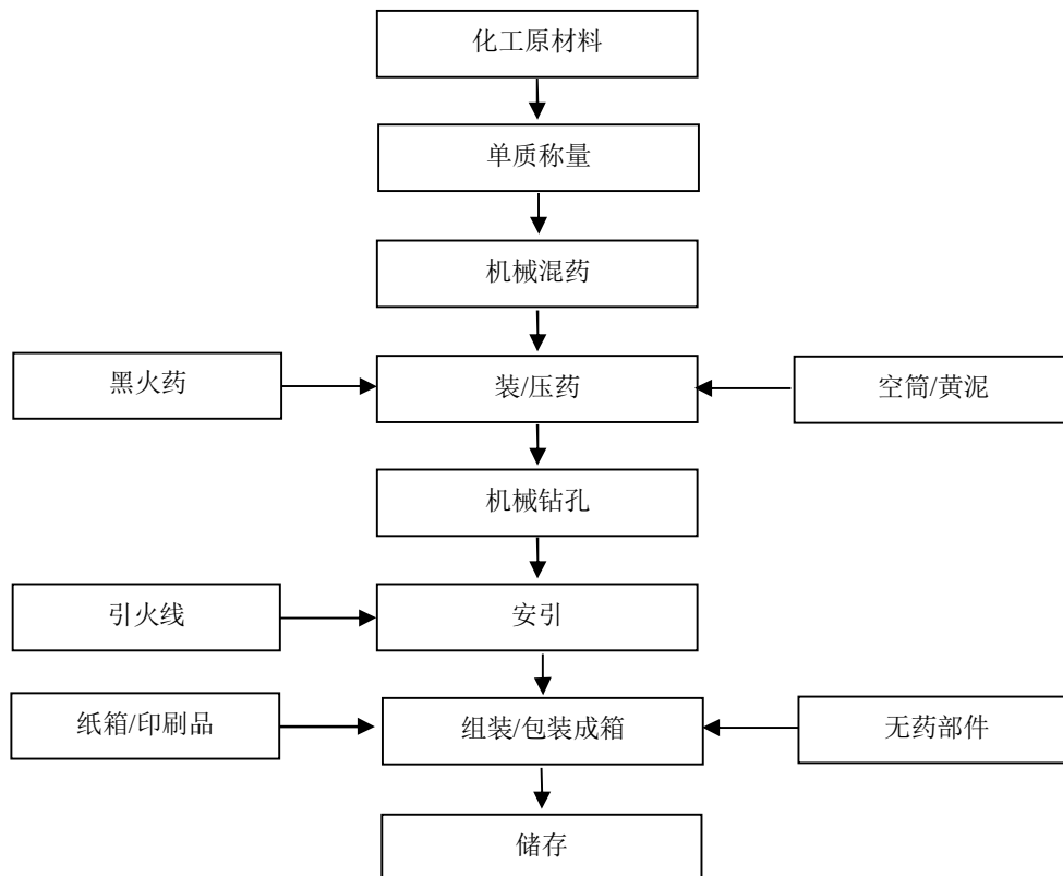
图 2-3：升空类（旋转升空烟花）/旋转类（大地花开）生产工艺流程图
