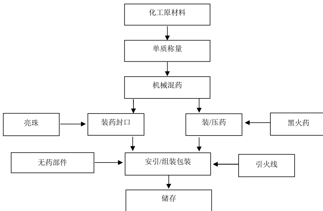
图 2-2：升空类（火箭）生产工艺流程图
