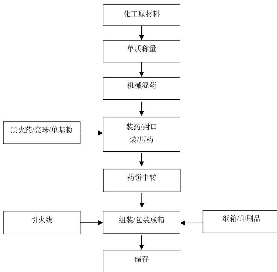
图 2-1：喷花类/玩具类（玩具造型）/组合烟花（喷花效果同类组合）生产工艺流程图
