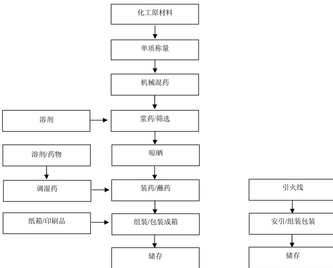
图 2-5：玩具类（线香型-晨光花）生产工艺流程图
