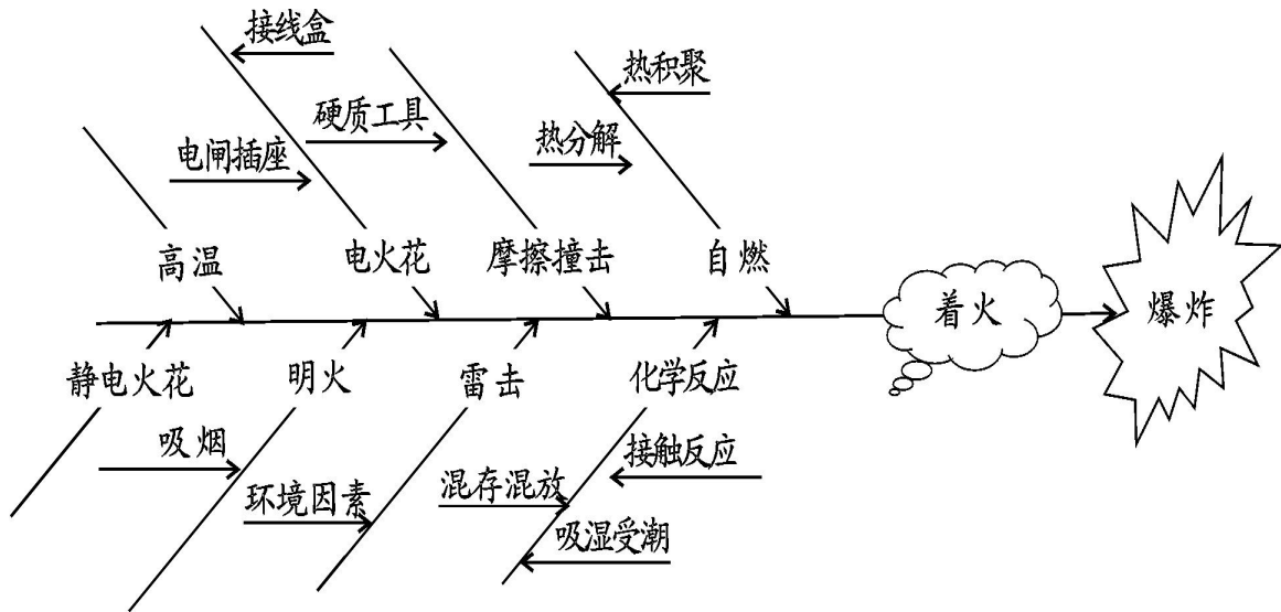
图 3-1 烟花爆竹仓库引爆的原因分析图
