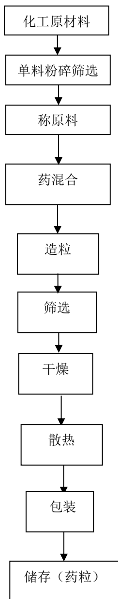
图 2-4-1 亮珠生产流程图
