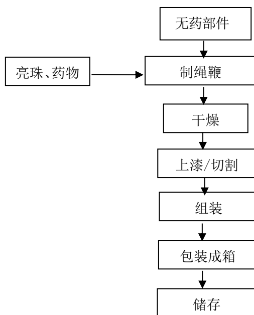
图 2-4-3 玩具类（线香型/绳鞭）生产工艺流程图
