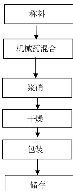
图 2-4-2 制硝生产工艺流程图
