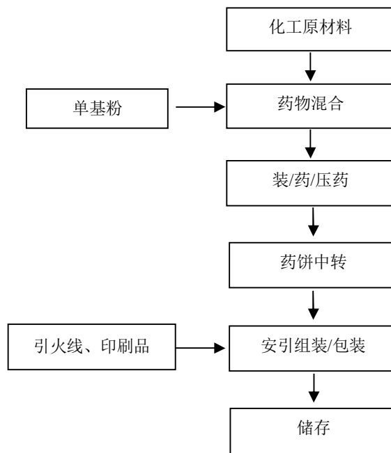
图 2-3：喷花类生产工艺流程图
