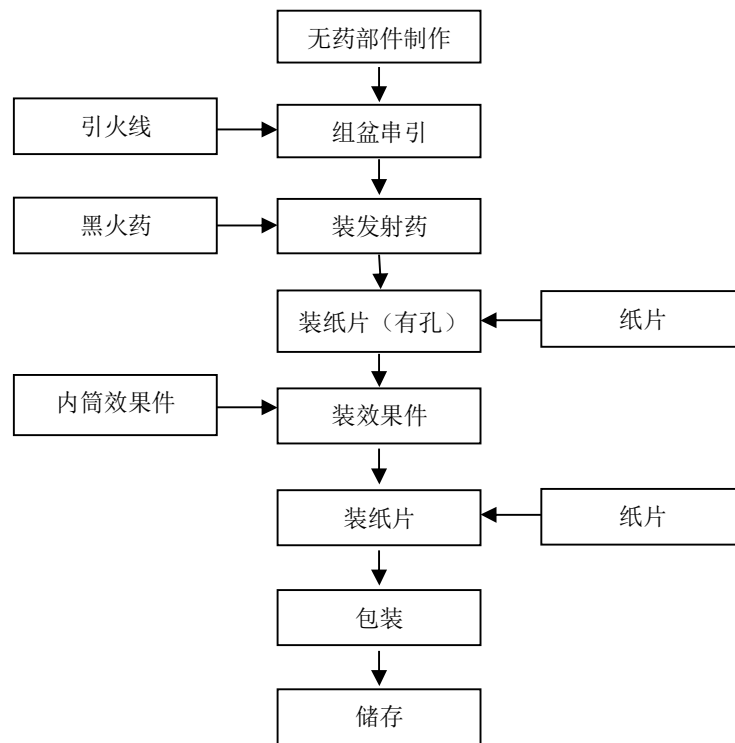
图 2-1：组合烟花生产工艺流程图
