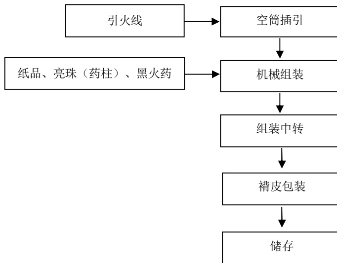
图 2-4：吐珠类生产工艺流程图
