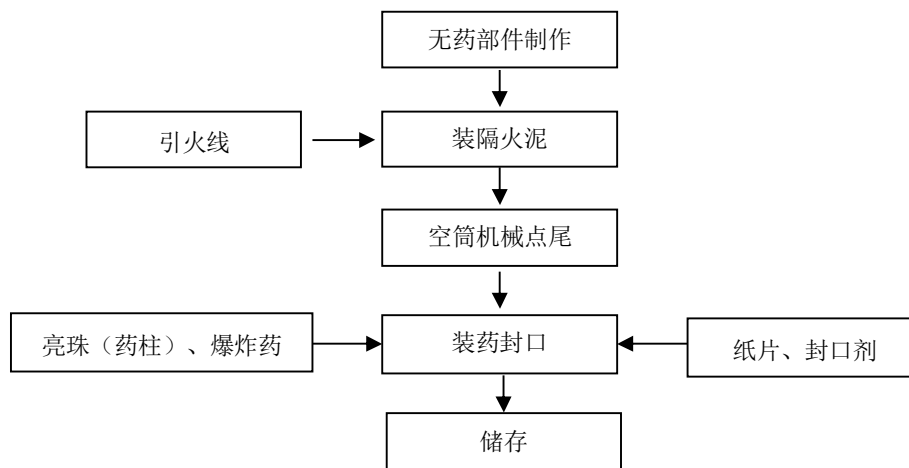
图 2-2：效果内筒生产工艺流程图
