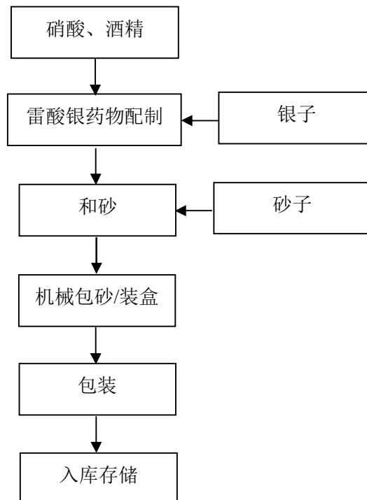
图 2-1 砂炮生产工艺流程图
