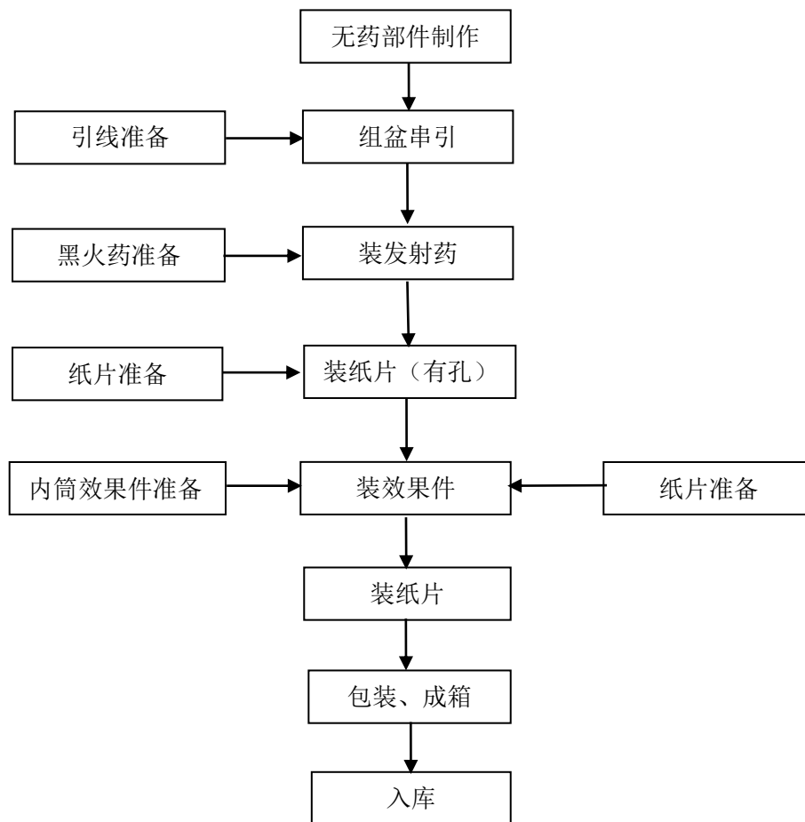
图 2.4-3 组合烟花类产品生产工艺流程图
