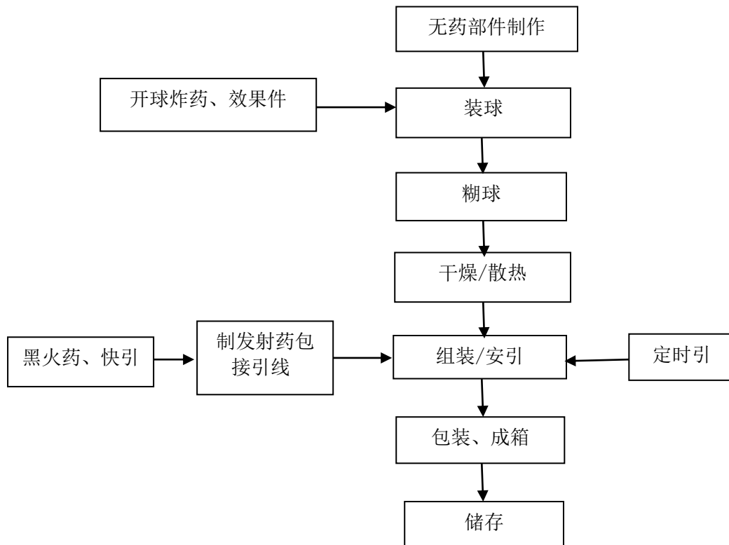
图 2.4-4 礼花类（小礼花）产品生产工艺流程图
