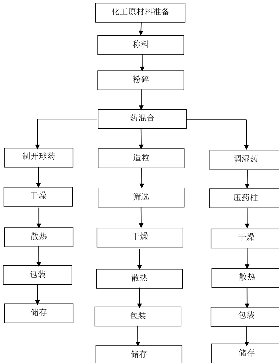
2.4-1 亮珠、开球药、药柱生产工艺流程图
