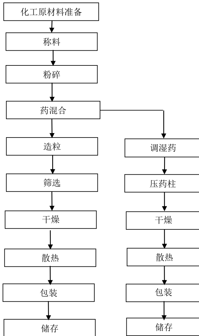
2.4-1 亮珠、药柱生产工艺流程图
