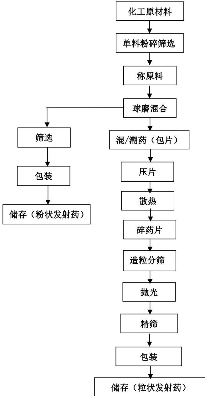
2-4-1 黑火药制造工艺流程图 (粉状、粒状发射药)
