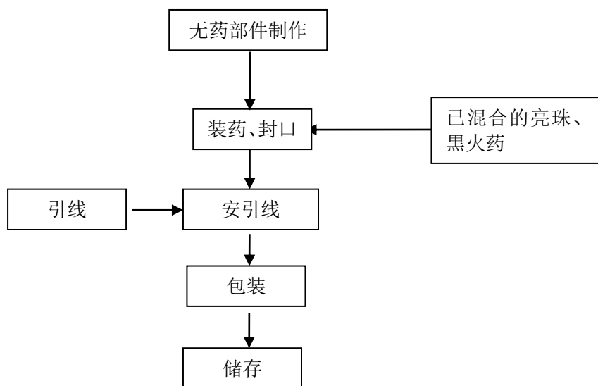
图 2.6-4 喷花类产品生产流程图
