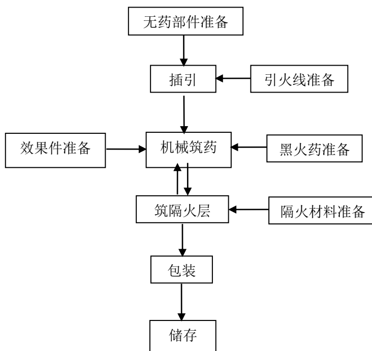
图 2.6-5 吐珠类产品生产工艺流程图
