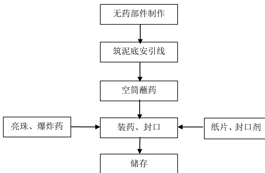
图 2.6-2 效果内筒生产工艺流程图
