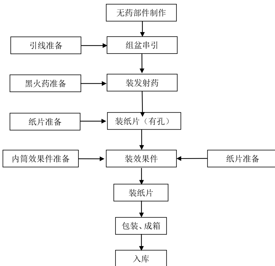
图 2.6-3 组合烟花类产品生产工艺流程图
