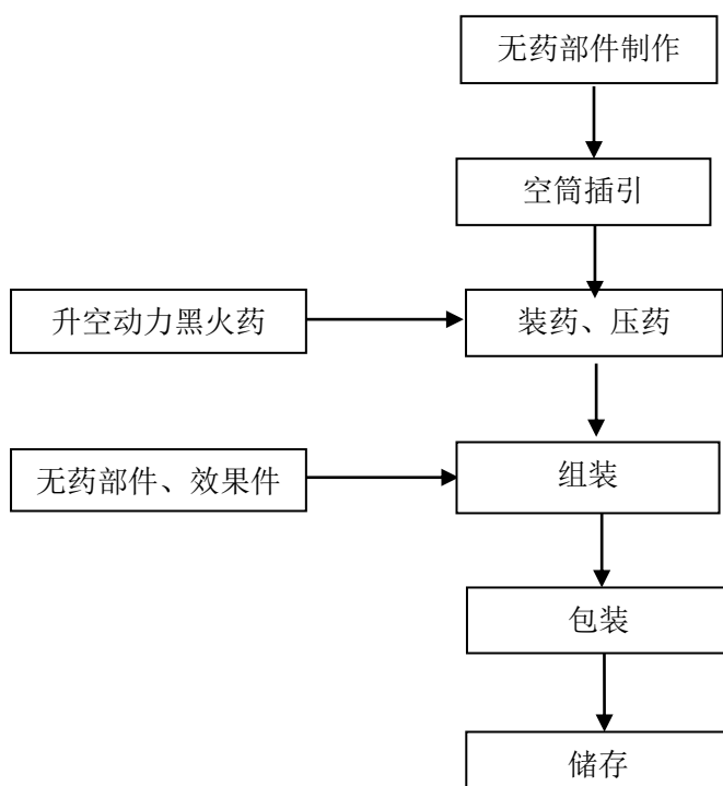
图 2.4-3 升空类（小型火箭）产品生产工艺流程图
