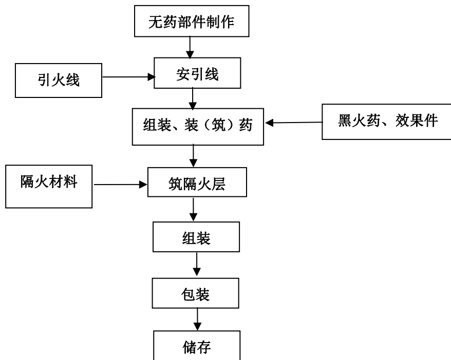
图 2-4-4 吐珠类产品生产工艺流程图
