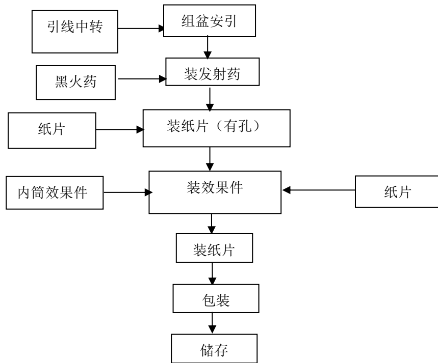
图 2-4-3 组合烟花产品生产工艺流程图
