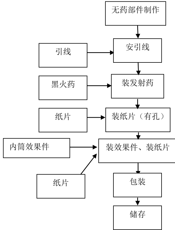
图 2.4-5 小礼花生产工艺流程图
