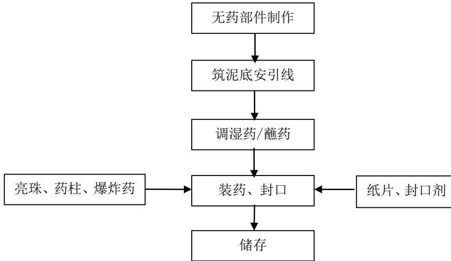
图 2.4-1 效果内筒生产工艺流程图
