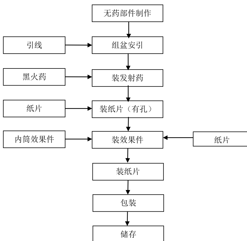
图 2.4-3 组合烟花生产流程图
