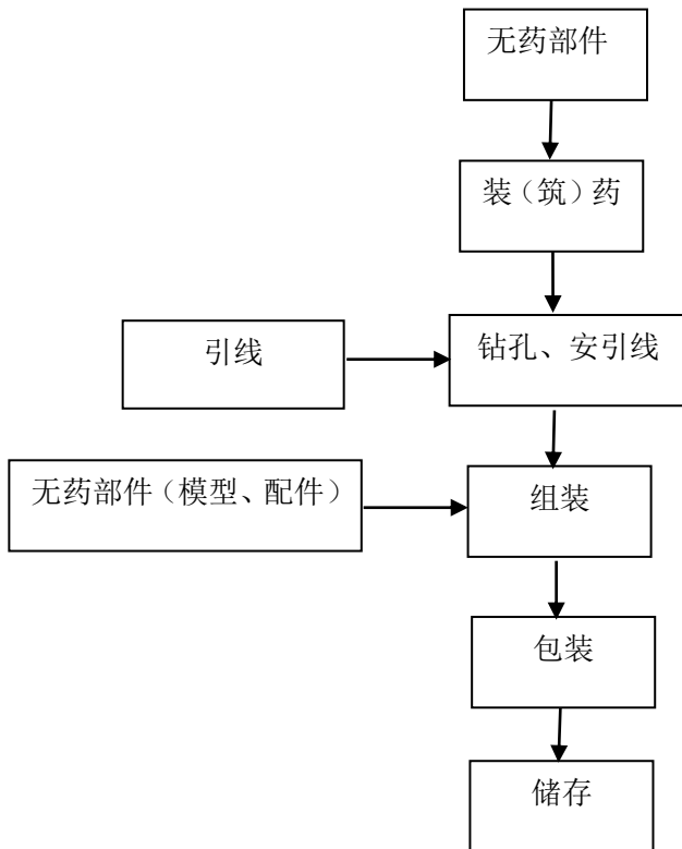
图 2.4-6 玩具类（玩具造型）产品生产工艺流程图
