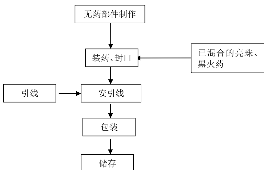
图 2.4-3 组合烟花生产流程图
