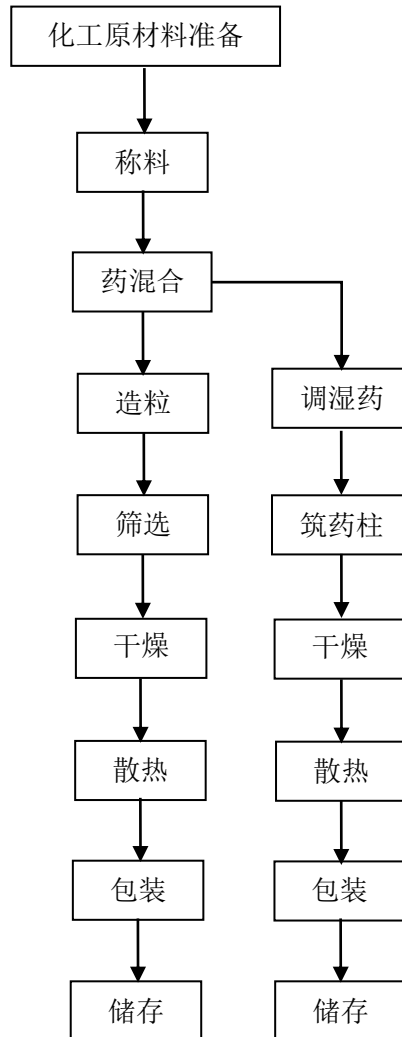
图 2.4-2 亮珠、药柱生产工艺流程图
