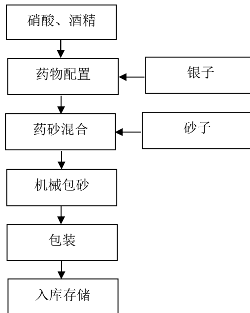
图 2-4：玩具类（摩擦型-砂炮）生产工艺流程图
