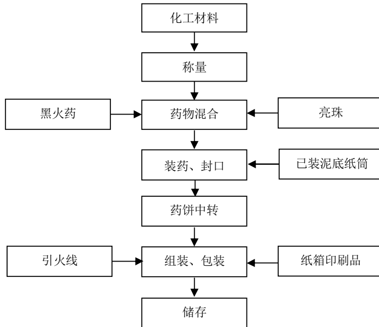
图 2-1：组合烟花（喷花）生产工艺流程图
