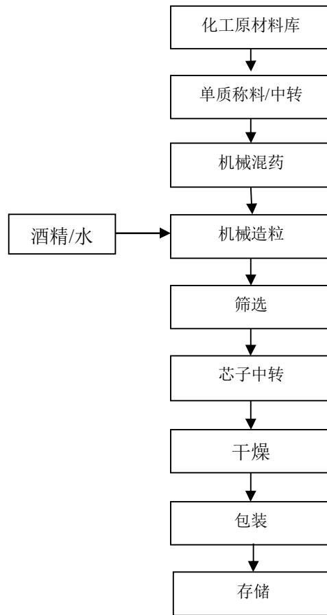
图 2-3：亮珠生产工艺流程图
