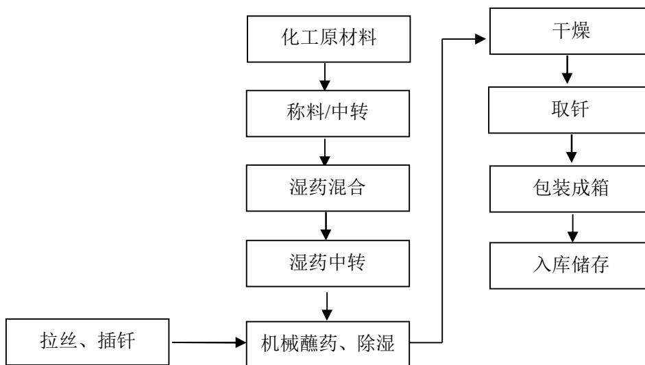
图 2-2：玩具类（线香型-电光花）生产工艺流程图
