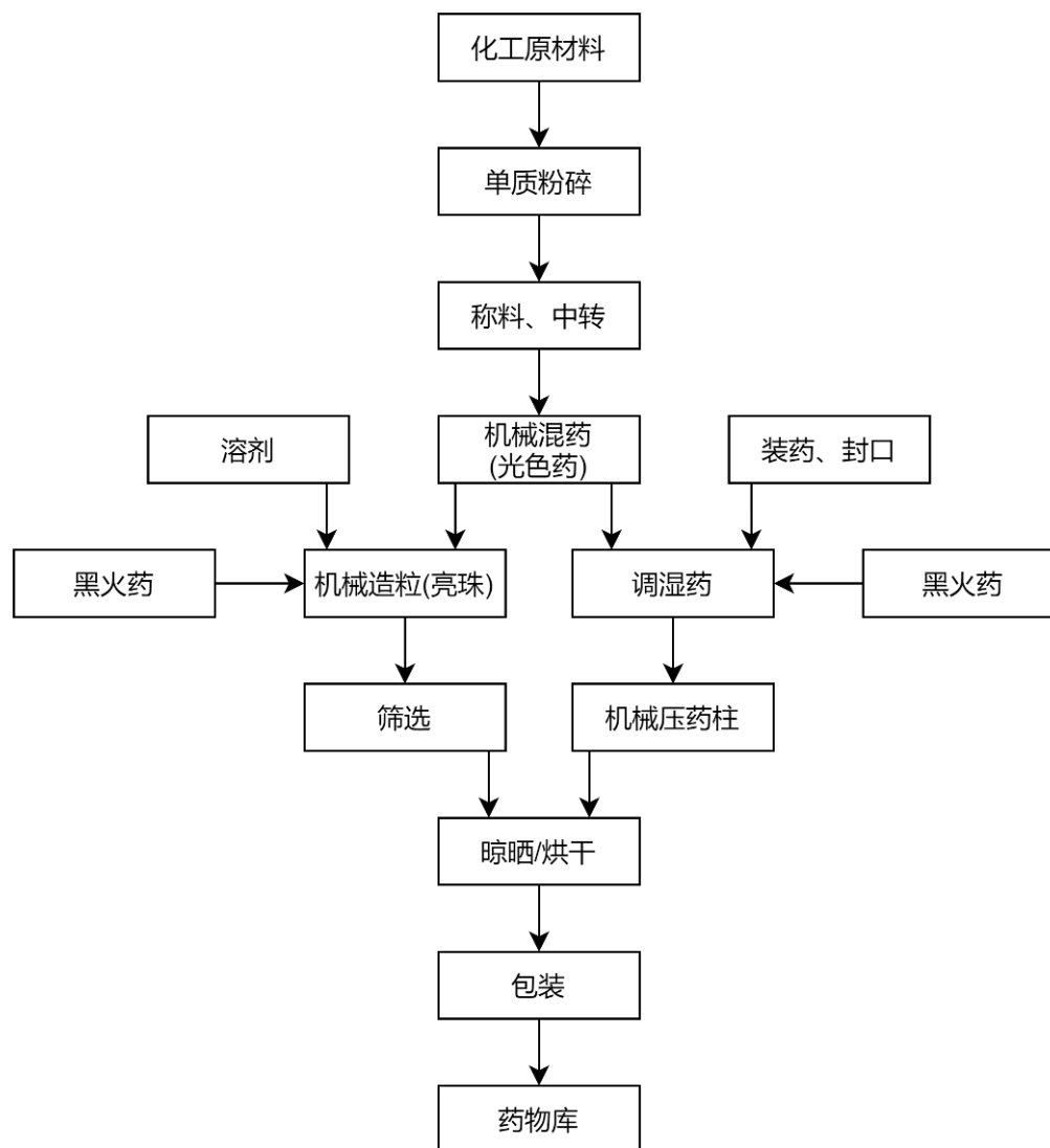
图 2-3：烟火药（亮珠/药柱）工艺流程图
