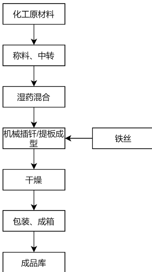
图 2-2：D 级玩具类（线香型）工艺流程图
