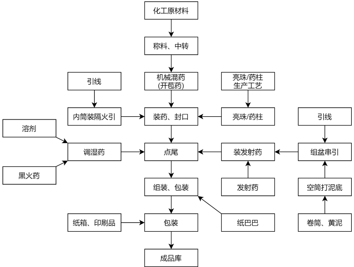
图 2-1：C 级组合烟花类工艺流程图
