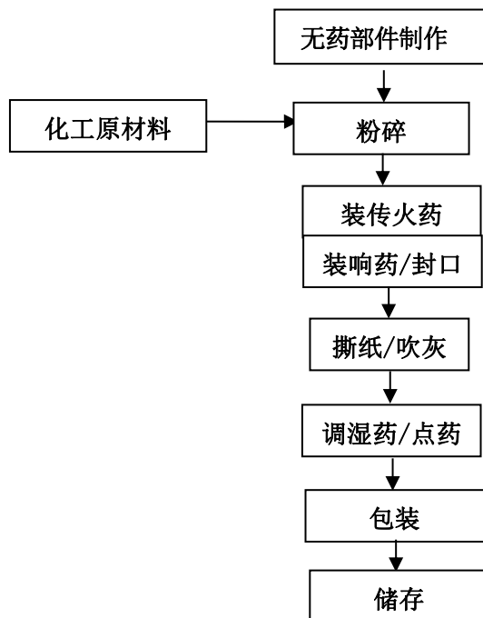
图 2-4-1 爆竹类（擦炮）生产工艺流程图
