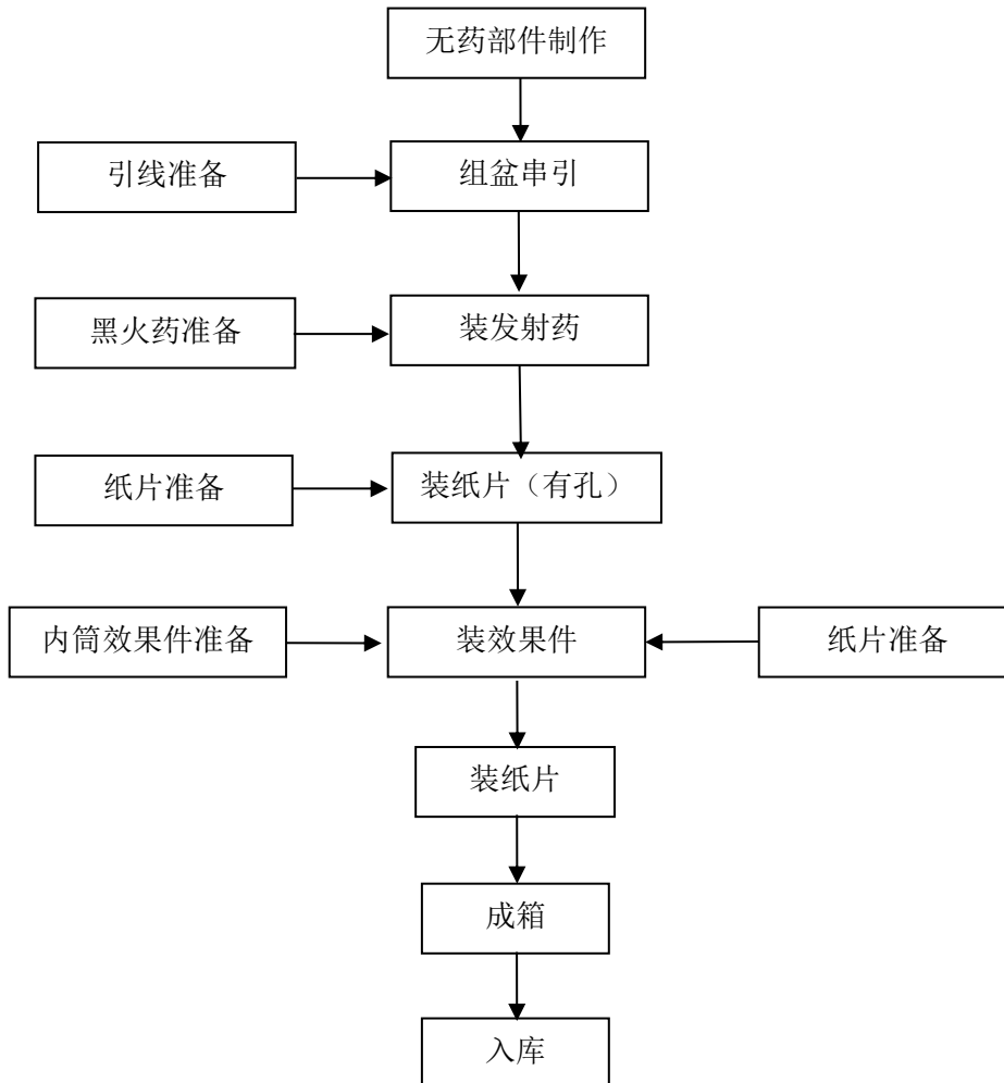
图 2.4-3 组合烟花类产品生产工艺流程图
