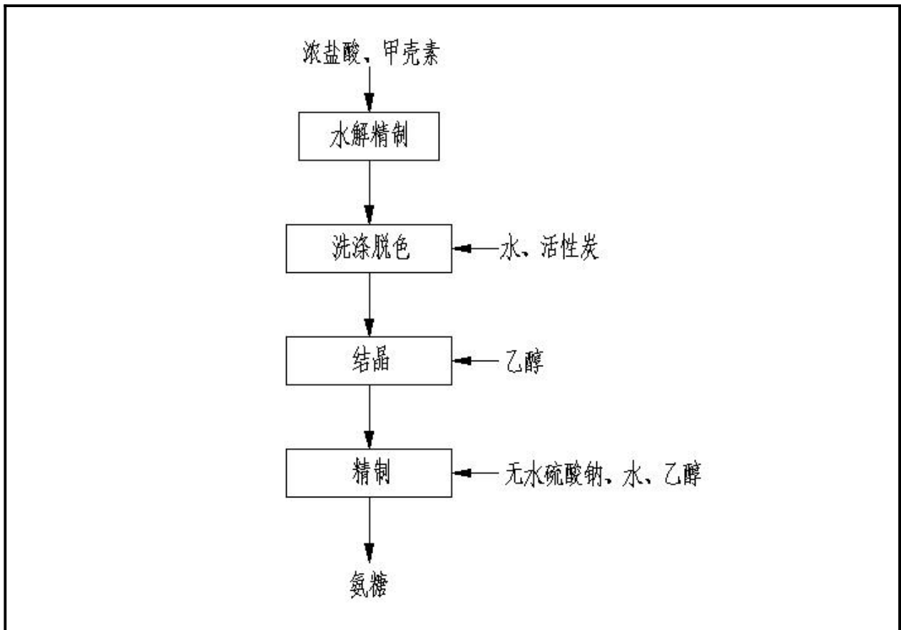
图 2.4.1.2-6 氨基糖（位于 B06 三车间）生产工艺流程图
